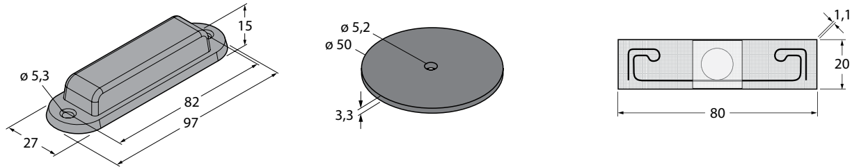
Fig. 15: BL ident® UHF tags (examples)
